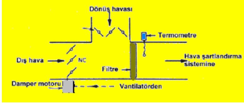
Şekil 2.1: Minimum dış hava damperi çalışma şeması
