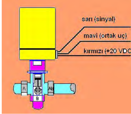
Şekil 2.5: Hidrolik operatör
