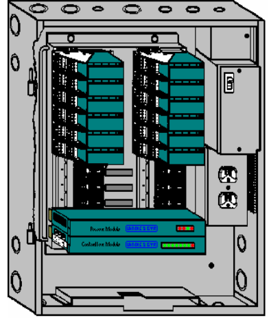
Şekil 3.6: Saha bilgisayarı (PLC)
