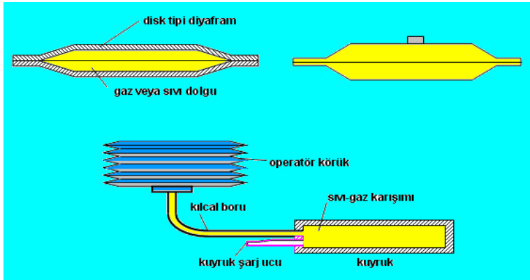
Şekil 1.2: Contalı ve körük eleman hissedici tipleri
