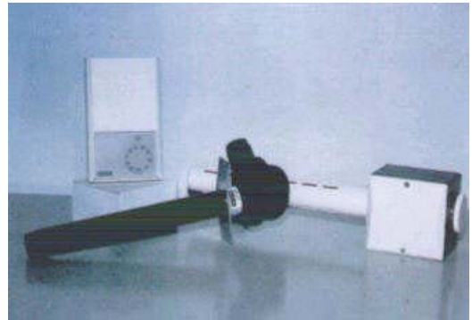
Resim 1.14: Çeşitli nem duyargaları
