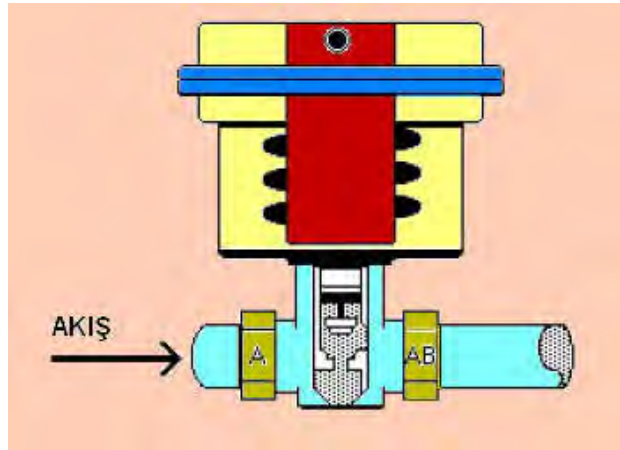
Şekil 2.4: Pnömatik operatör
