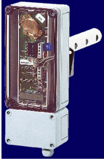
Resim 1.42: Kanal tip CO2 hissedici
