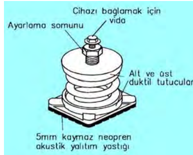
Şekil 5.2: Sismik sınırlayıcı yaylı takoz
