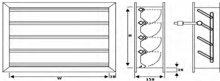
Şekil 2.3: Hava damperi görünüşleri
