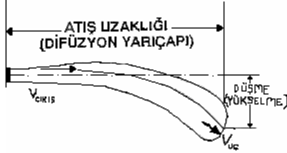
Şekil 2.2: Menfezin hava atış uzaklığı ve düşmesi
