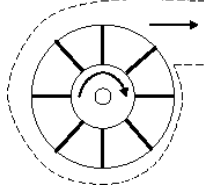
Şekil 1.4: Radyal (eğimsiz) tip
