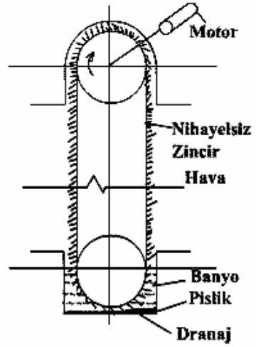
b) Temizlenir tip
