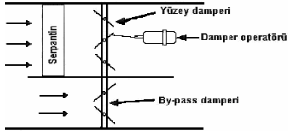
Şekil 2.5: Yüzey ve by-pass damperleri
