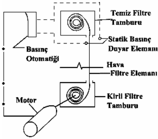
a) Atılır tip
